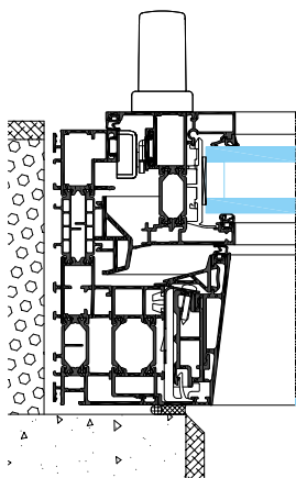
Vaakaleikkaus – pilotettu karmirakenne
