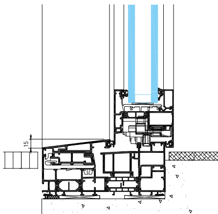
Pystyleikkaus – ovilehden kohta, matala kynny
