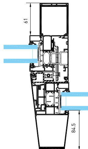
Vahvistettu keskilukitusprofiili
